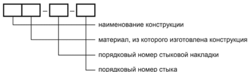
Рисунок А.2 - Условное обозначение блоков
