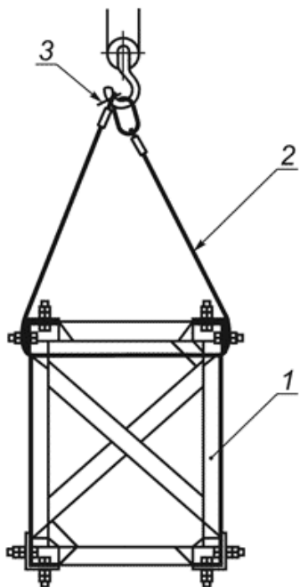
Рисунок Г.1 - Схема монтажа ригелей с расчетной длиной 17,0 м
