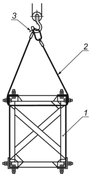
Рисунок Г.3 - Схема монтажа ригелей с расчетной длиной 34,0; 39,0; 44,0; 55,5 и 64,5 м
